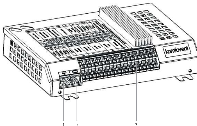
Obr. 1.3a. Řídící jednotka s připojovacími svorkami
