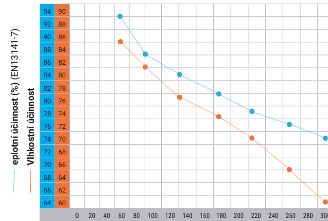
ÚČINNOSTNÍ GRAF XHOUSE-300 - ERV
