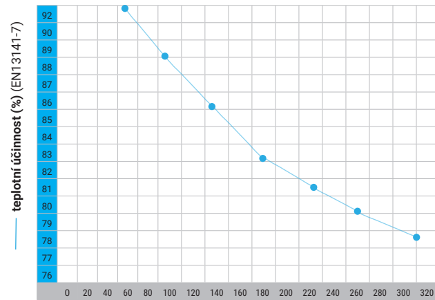
ÚČINNOSTNÍ GRAF XHOUSE-300 - HRV
