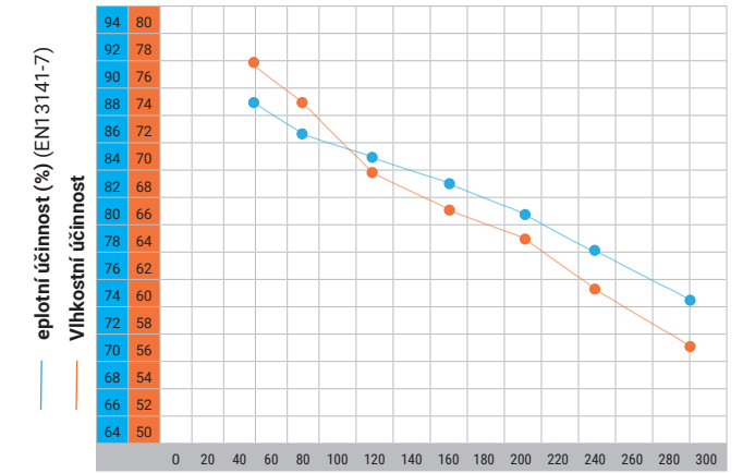
ÚČINNOSTNÍ GRAF XHOUSE-300 - ERV
